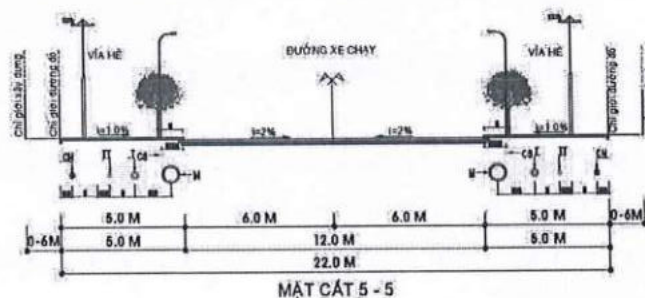
Hình 21. Mặt cắt giao thông 5-5 lộ giới 22m
