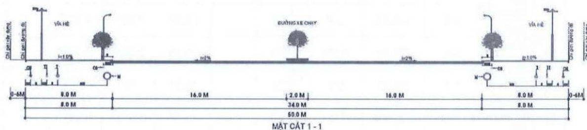
Hình 17. Mặt cắt giao thông 1-1 lộ giới 50m
