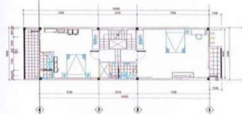
MẬT BẢNG LẤU 23.4.5 TL: 1/100
