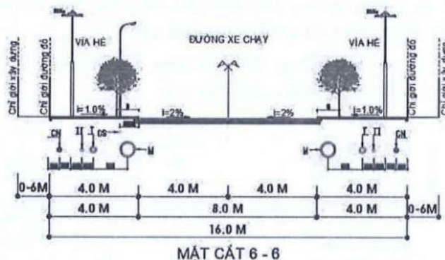
Hình 23. Mặt cắt giao thông 6-6 lộ giới 16m
