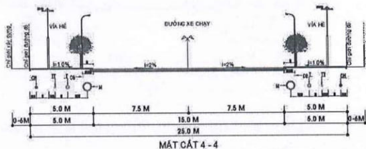
Hình 20. Mặt cắt giao thông 4-4 lộ giới 25m
