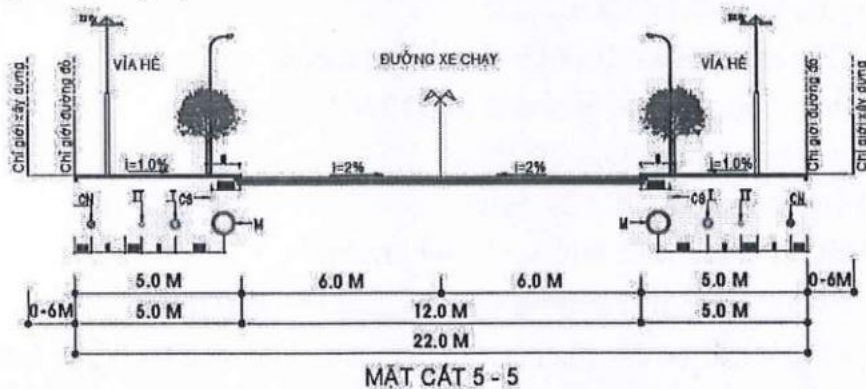
Hình 6: Mặt cắt giao thông 5-5 lộ giới 22m
