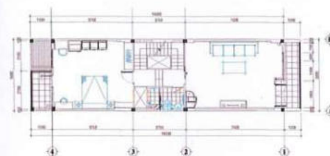
MẬT BẢNG LƯU 1 TL:1/90
