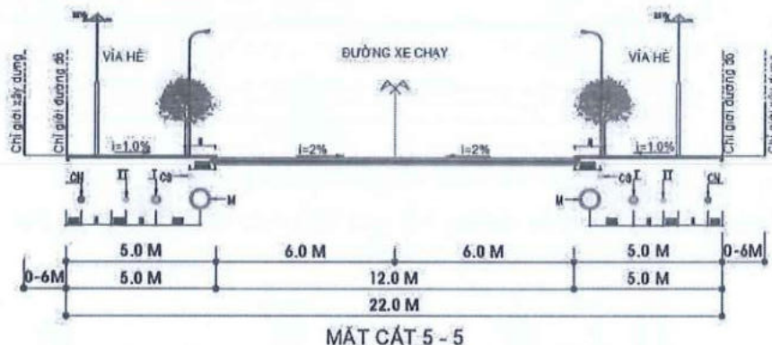
Hình 22. Mặt cắt giao thông 5-5 lộ giới 22m
