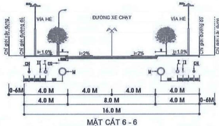
Hình 7: Mặt cắt giao thông 6-6 lộ giới 16m
