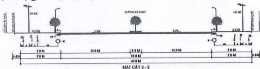
Hình 19. Mặt cắt giao thông 3-3 lộ giới 40m
