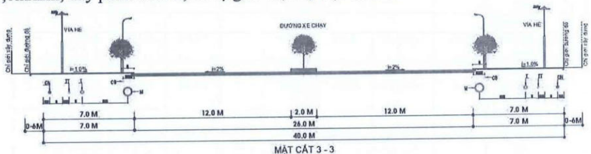
Hình 3: Mặt cắt giao thông 3-3 lộ giới 40m
