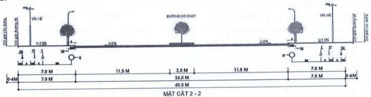
Hình 2: Mặt cắt giao thông 2-2 lộ giới 40m
