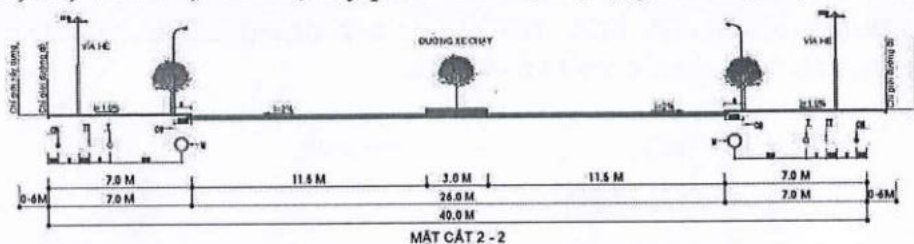
Hình 18. Mặt cắt giao thông 2-2 lộ giới 40m
