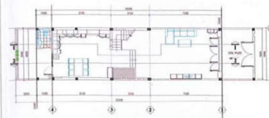
MẬT ĐĂNG TRỆT TL: 1/100
